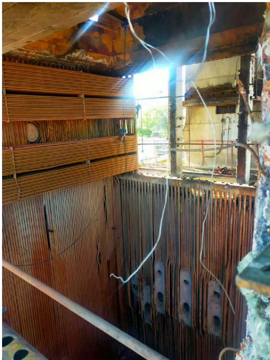
Водогрейный котел ПТВМ-100 ст.№3. КР котла с 100% заменой конвективных пакетов без коллекторов
