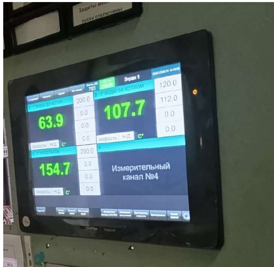
Регистратор многоканальный, технологический M/B/t0040/-/6;24/-/-/R/-/8/-/ГП/ТУ, PMT 59 /VG-10-230-P-1-0- B-0/8xUN-16xRO/PW8/v2.0-KZ/ЭлМетро-ВиЭР-104К-4АВ- 4АП-4ДВ
